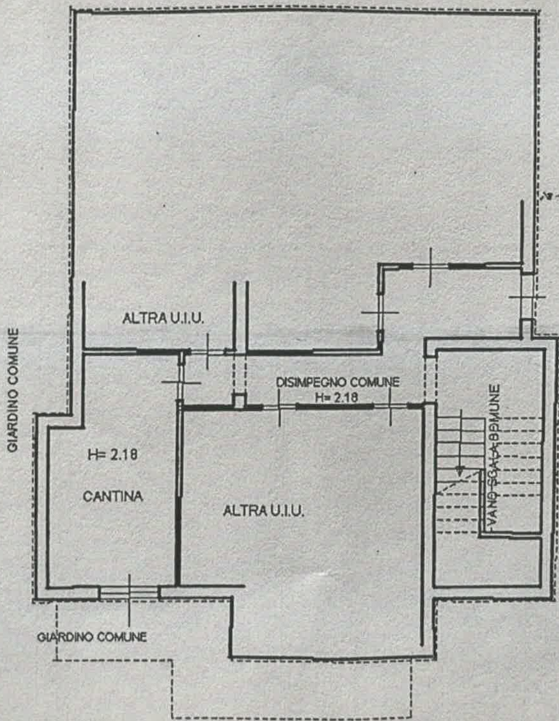
PIANO PRIMO SOTTOSTRADA
